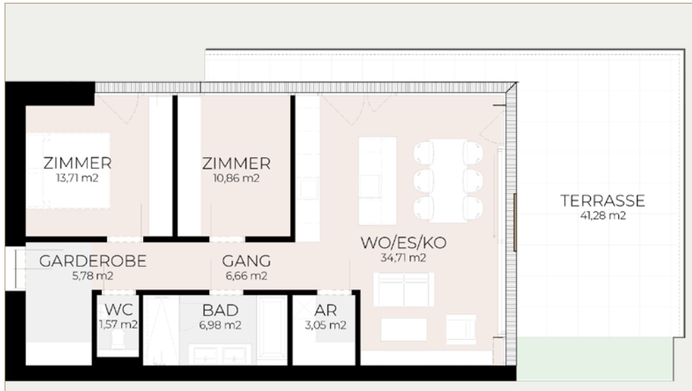
Wohnung 103 – 1. Obergeschoss
