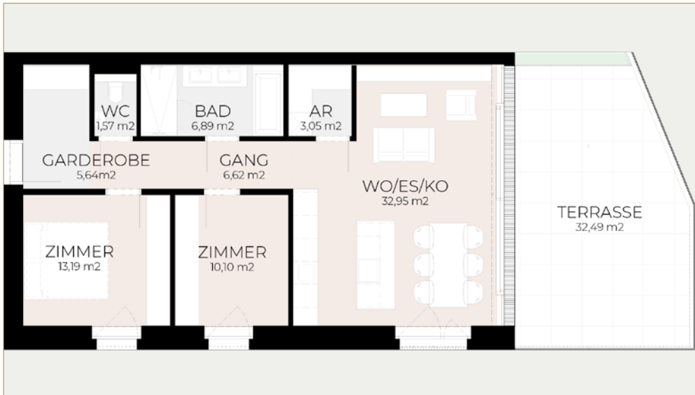
Wohnung 203 – 1. Obergeschoss
